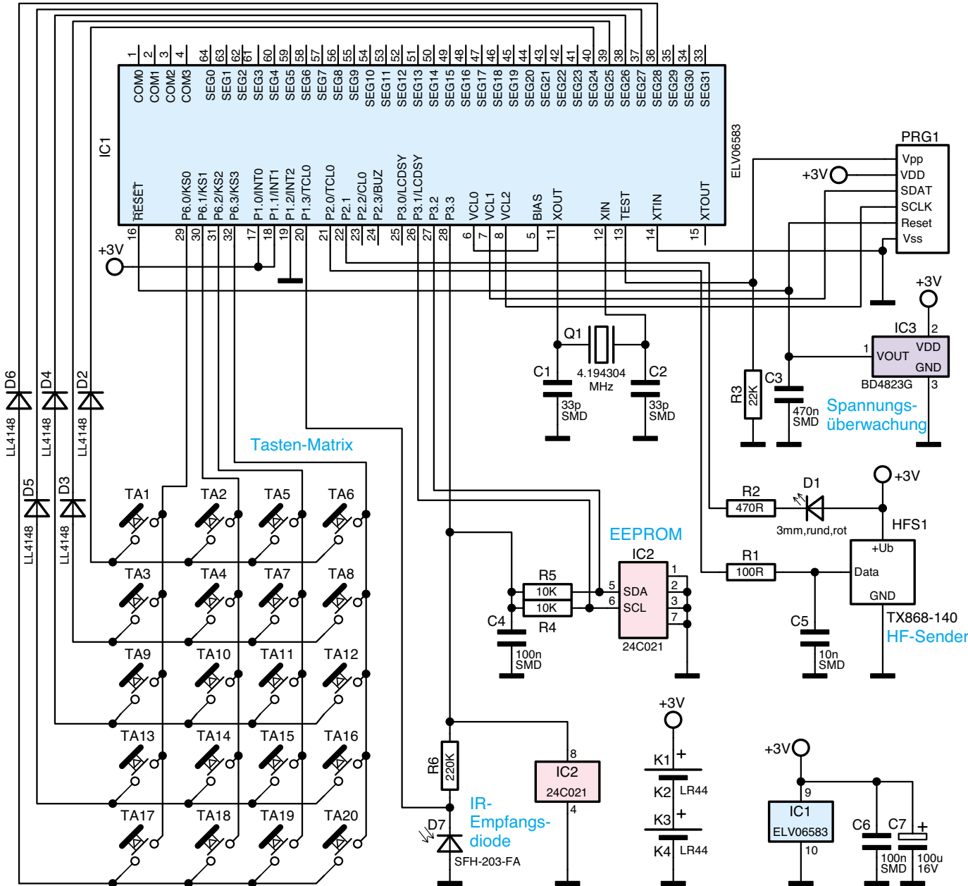
Bild 2: Schaltbild des Handsenders FS20 S20-3
