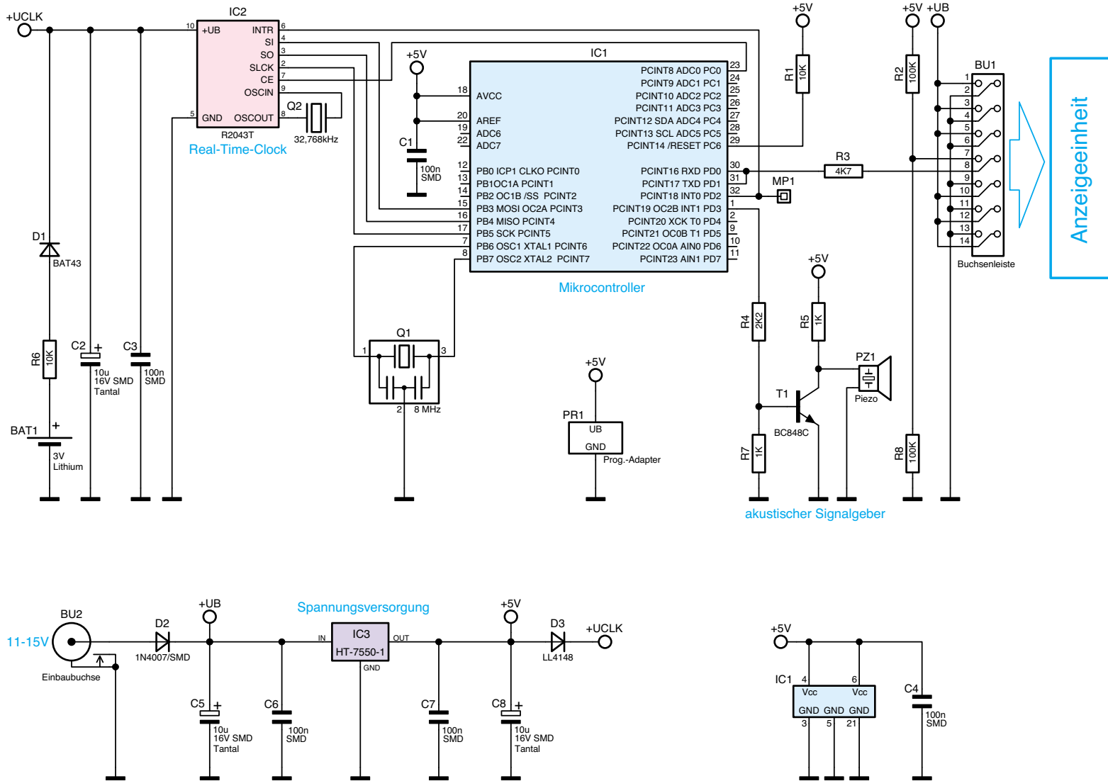
Bild 3: Die Schaltung der MFU 14. Die Anzeigeeinheit wird als fertig konfektionierte Baugruppe geliefert und ist deshalb nicht detailliert dargestellt.
