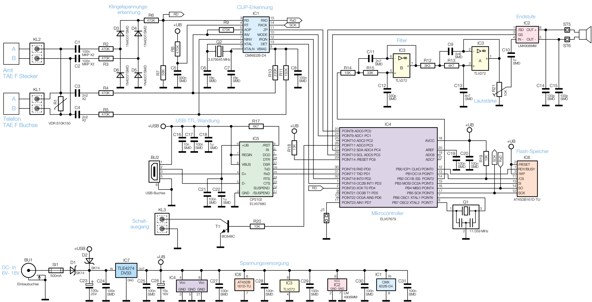
Bild 2: Das Schaltbild der CRE100
