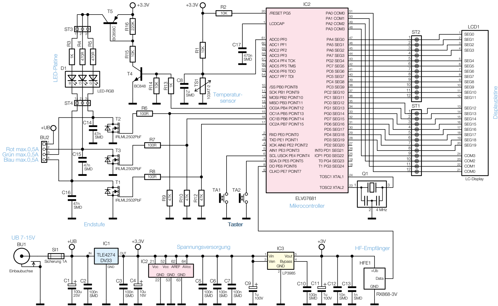
Bild 6: Schaltbild des WST 100
