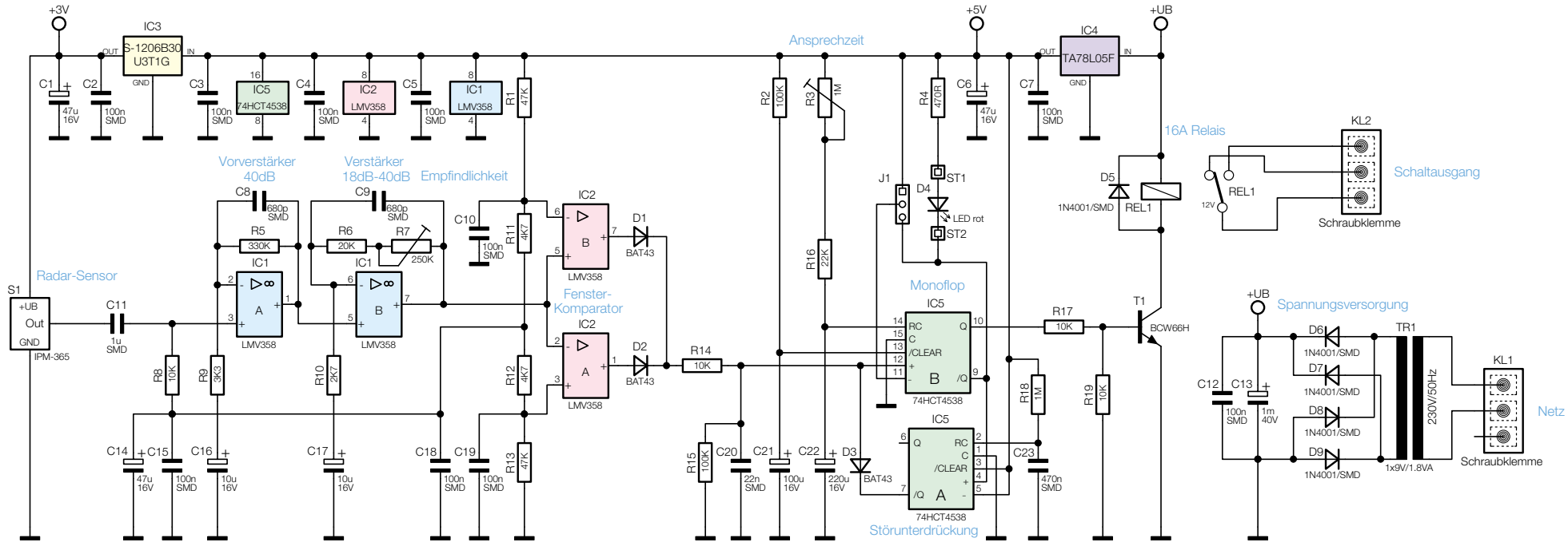
Bild 2: Schaltung des RBM 100
