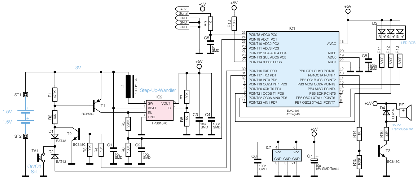
Bild 4: Schaltbild der Basisplatte
