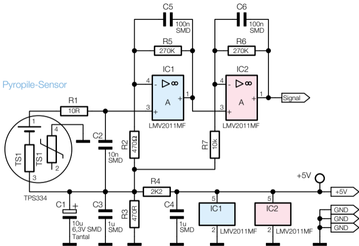
Bild 3: Schaltbild der Sensorplatte
