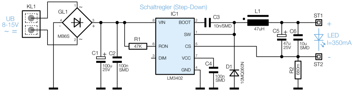
Bild 3: Schaltbild des LED12 AC
