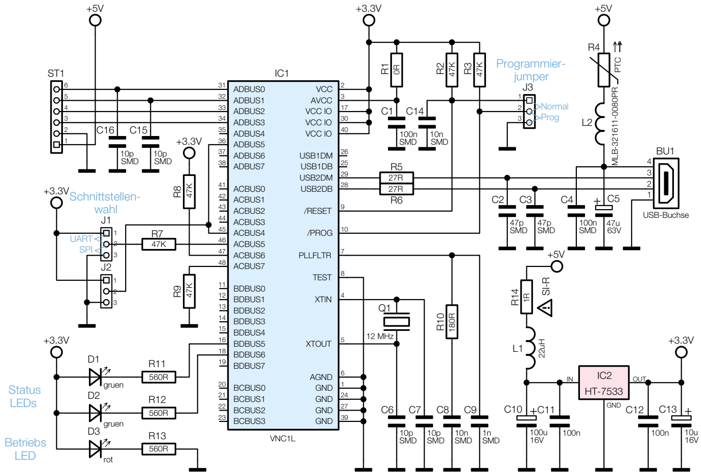
Bild 3: Schaltbild des ST1 100
