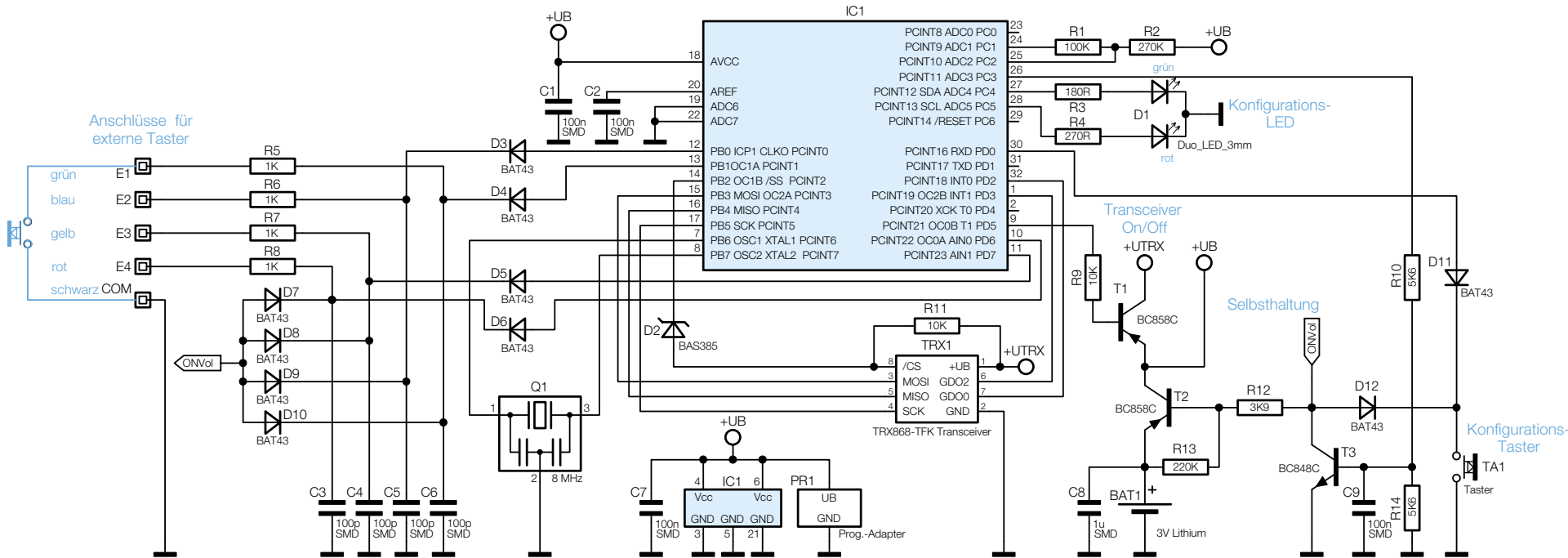
Bild 2: Schaltbild der Funk-Tasterschnittstelle HM-PBI-4-FM
