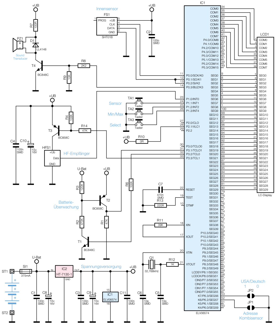
Bild 7: Schaltbild der WS 01
