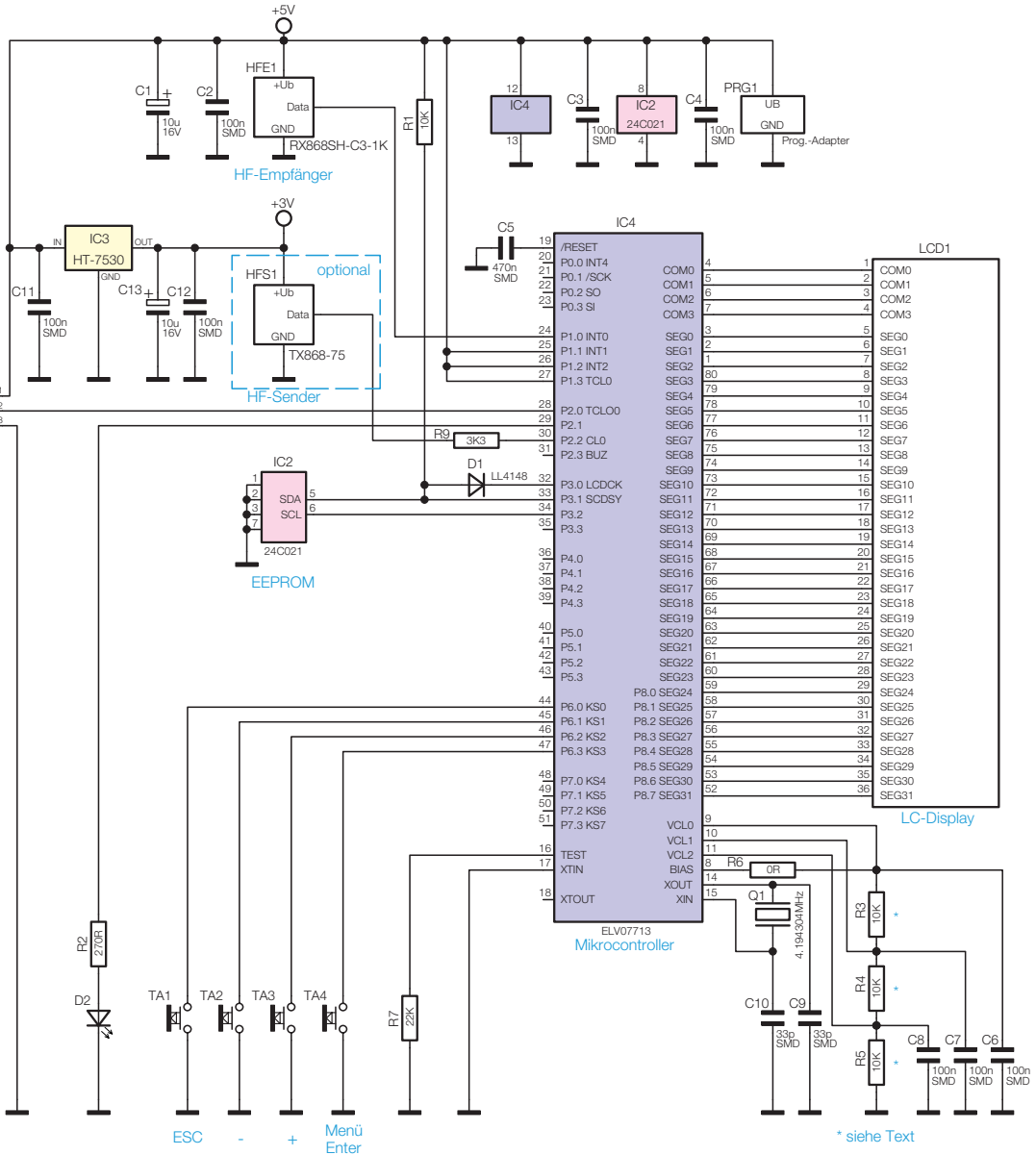
Bild 6: Die Schaltung des Controller-Teils mit Display, EEPROM und Sende-/Empfangsteil
