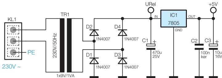
Bild 5: Die Schaltung von Netzteil, Schaltstufe und Relais-Schaltkontakt
