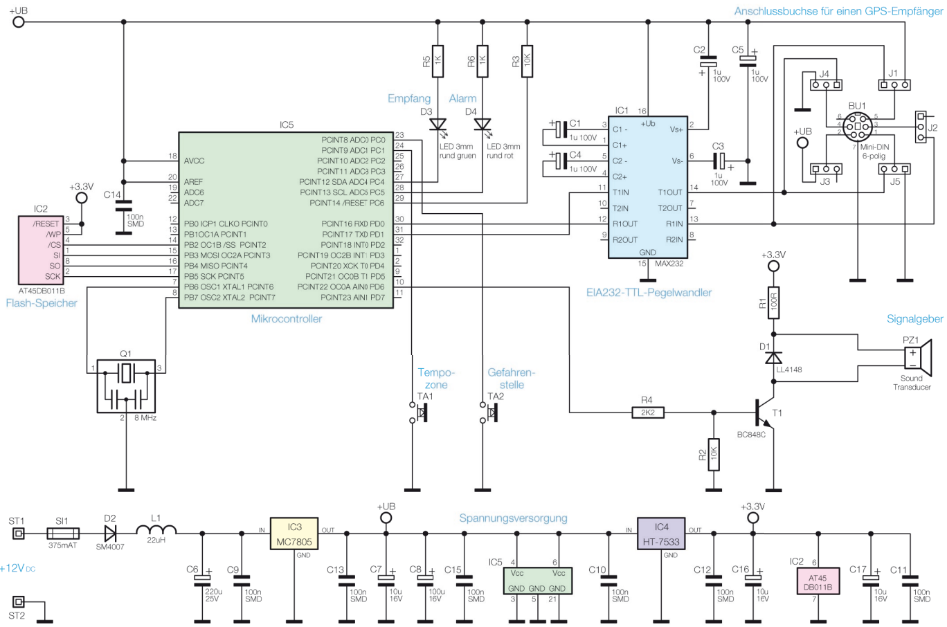
Bild 1: Die Schaltung des GPS-Gefahrenmelders
