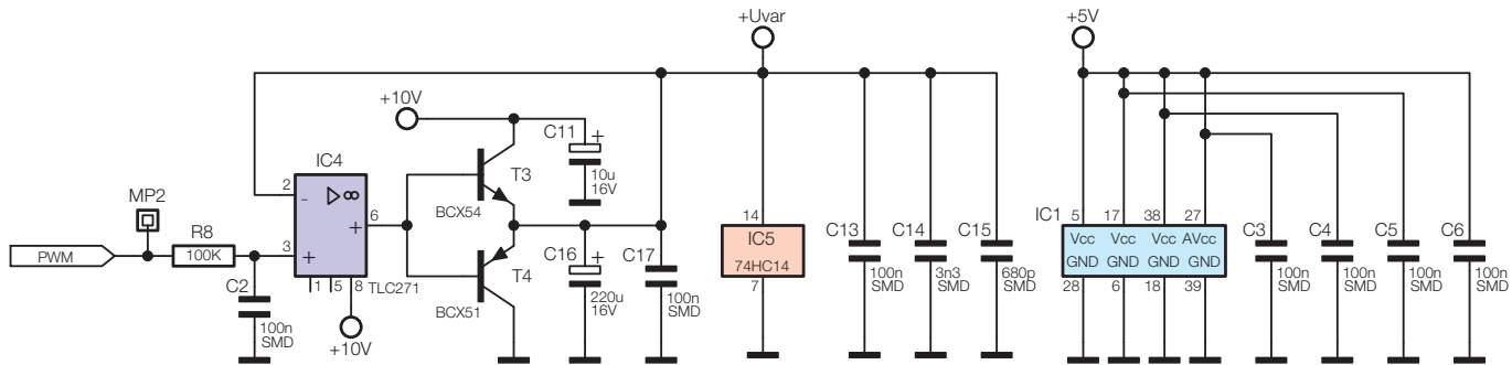
einstellbare Spannungsquelle
