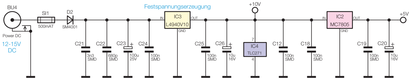
Bild 1: Die Spannungsversorgungen des UPG 100
