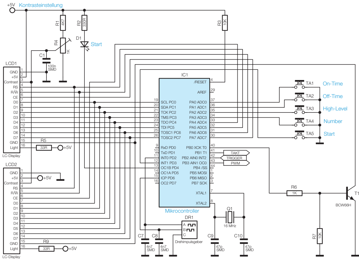
Bild 2: Die Mikrocontroller-Schaltung mit Bedienelementen und Anzeigen
