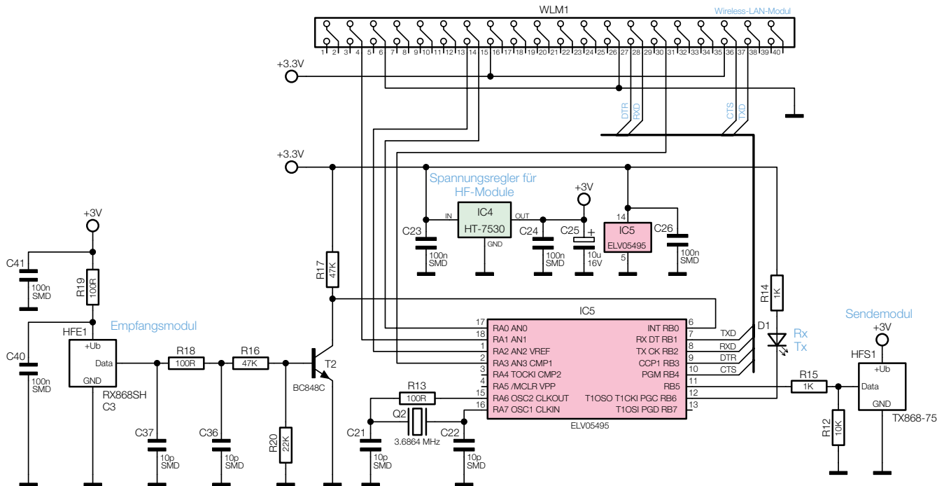
Bild 1: Schaltung der FHZ 1300 PC WLAN
