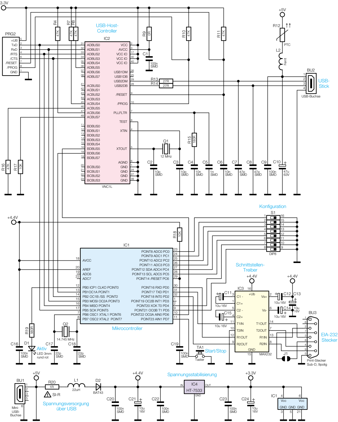
Bild 4: Das Schaltbild des SDU 1
