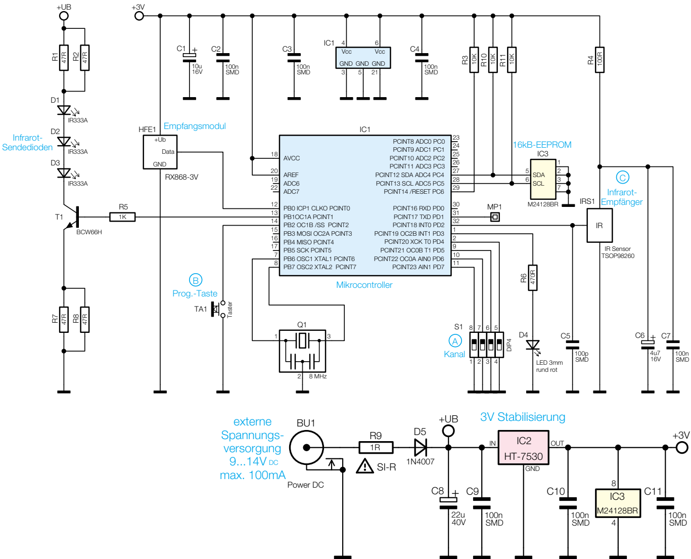
Bild 3: Schaltbild des FS20 IRF
