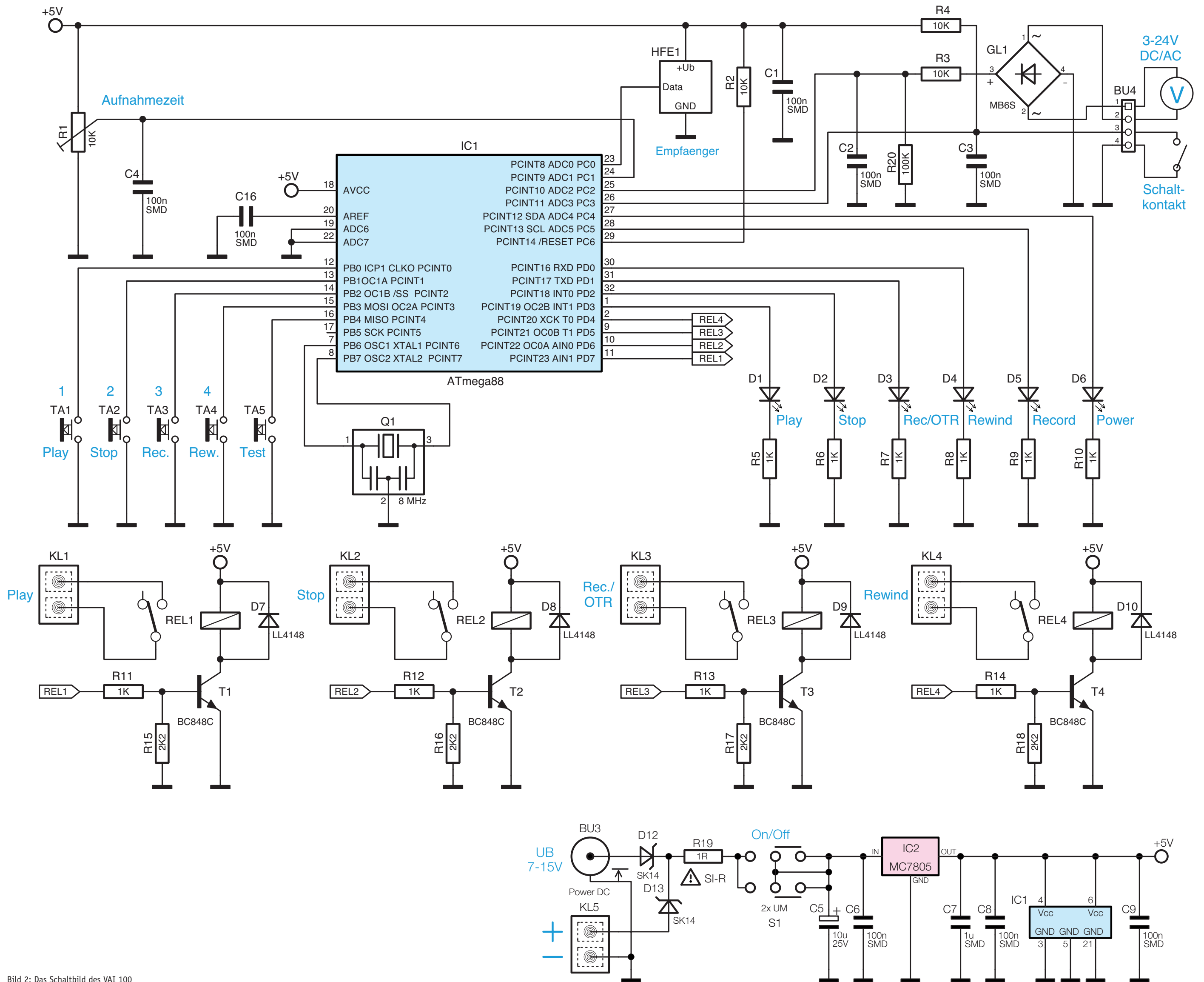
Bild 2: Das Schaltbild des VAI 100
