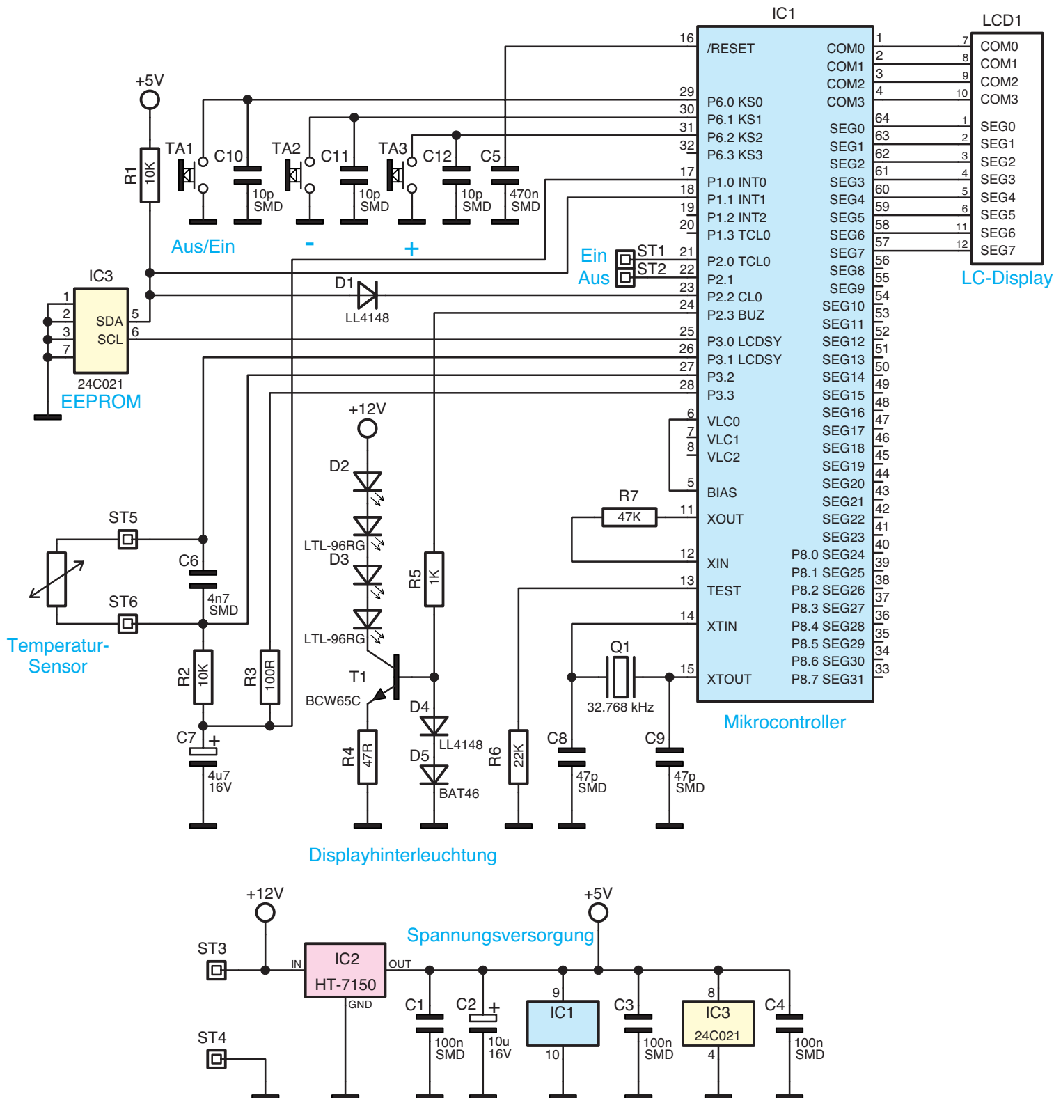
Bild 2: Die Hauptschaltung des UT 200
