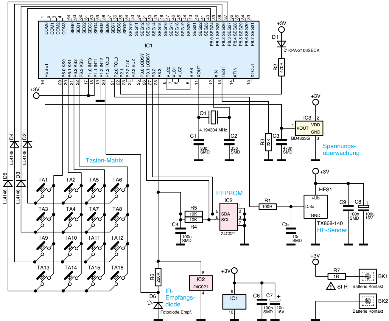
Bild 1: Das Schaltbild der FS20 S16
