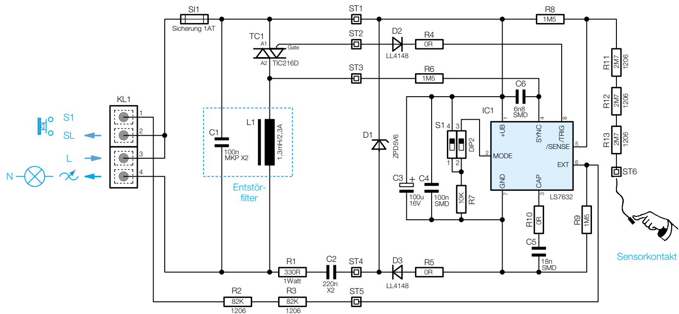
Bild 7: Die Schaltung des Phasenanschnittdimmers DI200 AN
