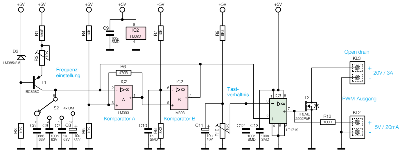
Bild 4: Die Schaltung des Pulsweiten-Modulators
