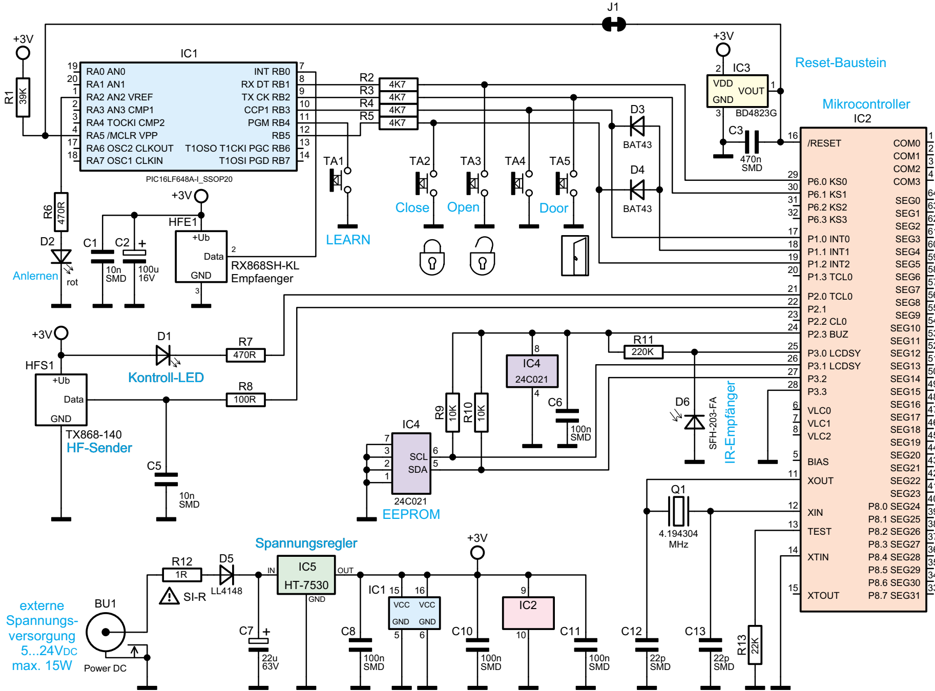
Bild 4: Schaltbild des KM300-FS20
