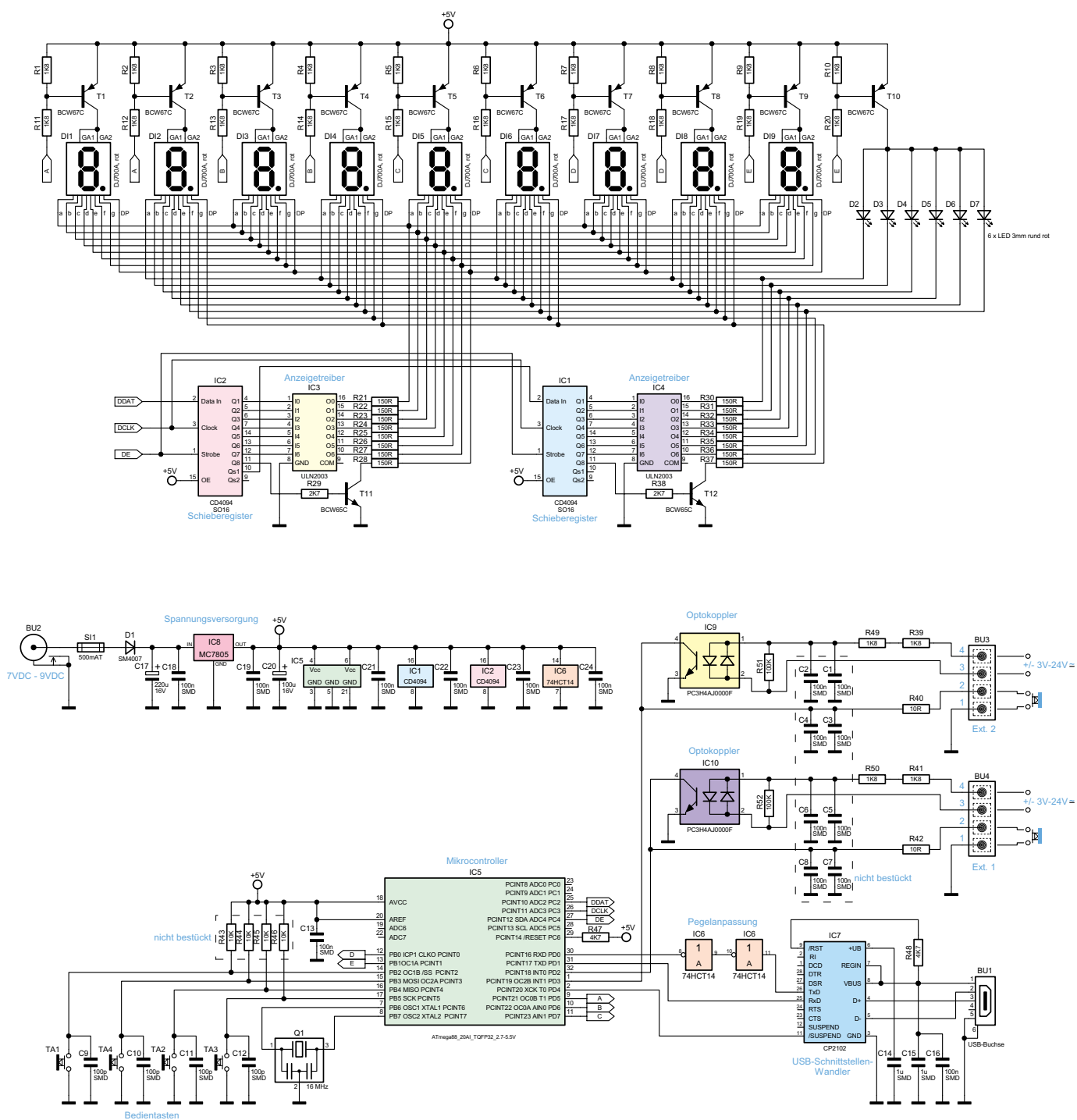
Bild 1: Das Schaltbild der LED-Stoppuhr LSU 100
