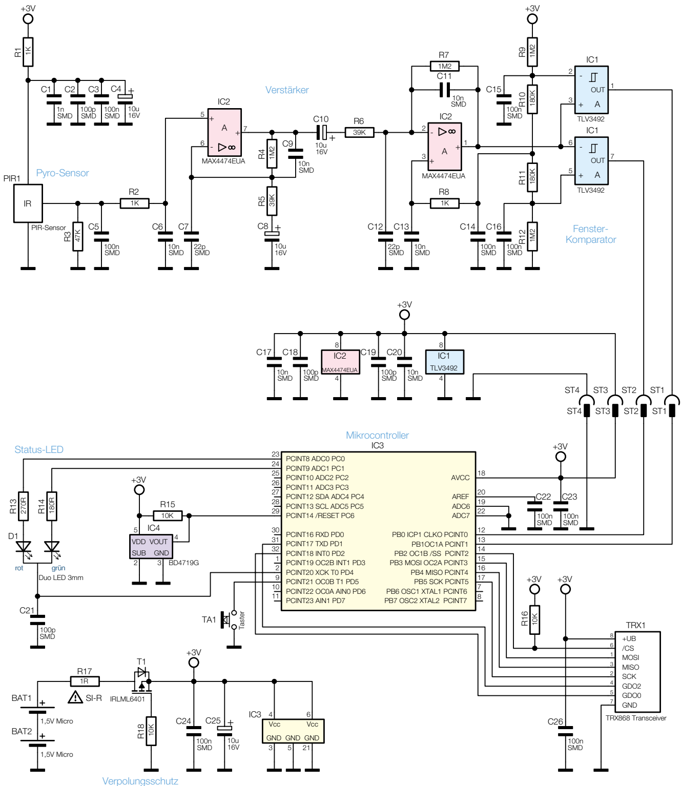
Bild 4: Die Schaltung des HM-Sen-MDIR-SM
