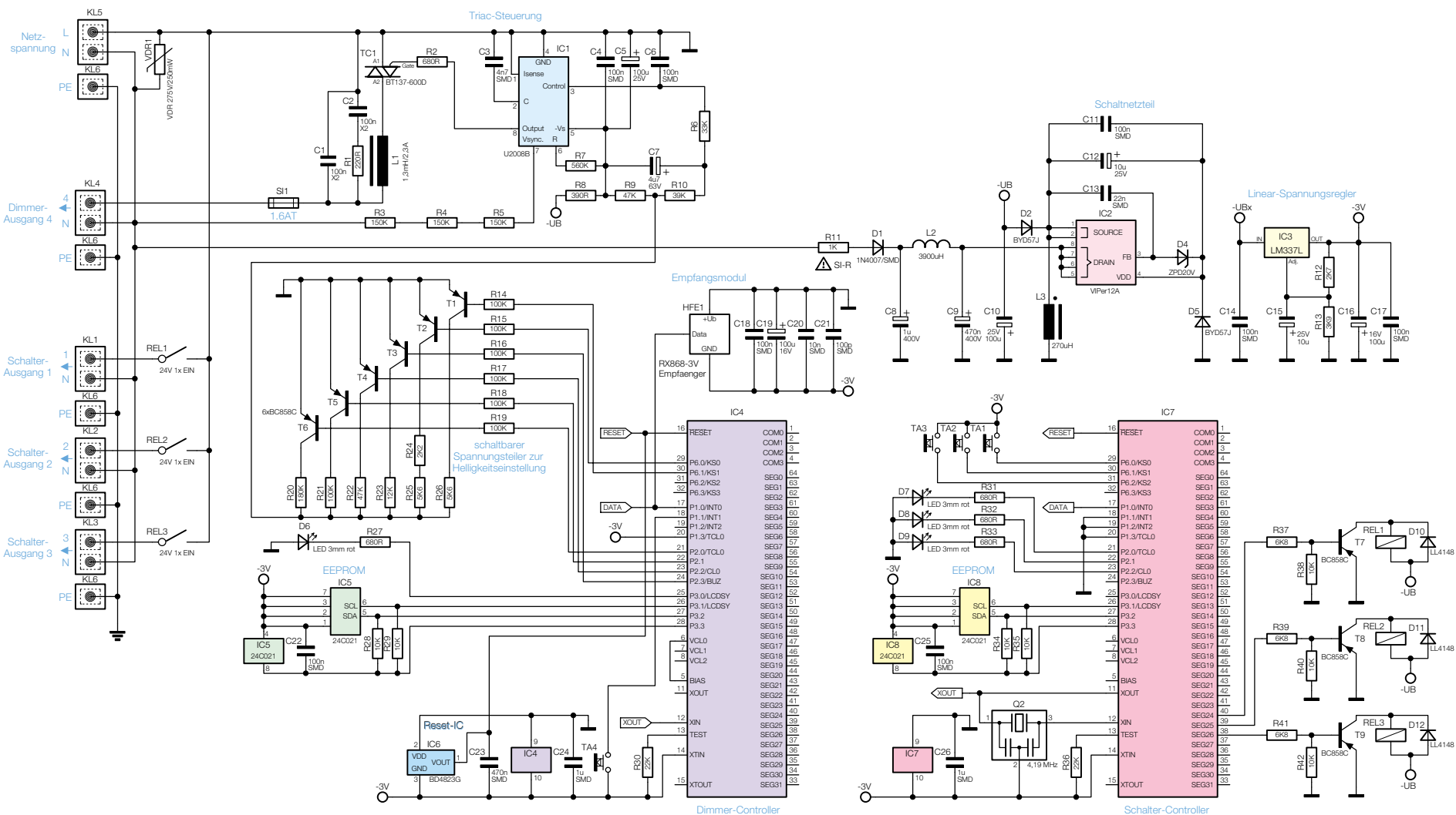
Bild 2: Die Schaltung des FS20 ASSD1
