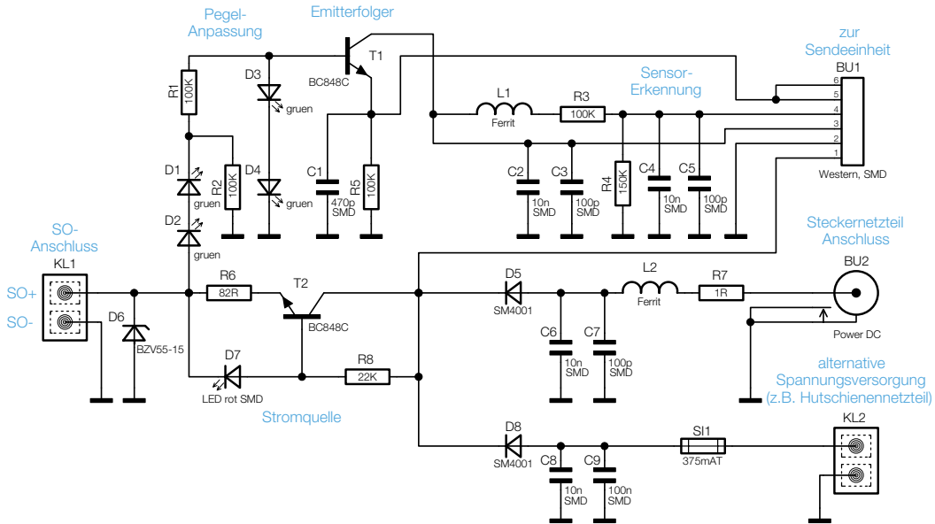
Bild 2: Schaltung des ESA 1000 WZ-SO
