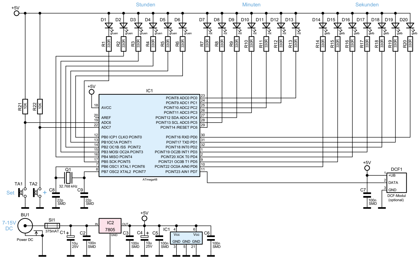
Bild 4: Die Schaltung der ELV-Binär-Uhr. Herzstück ist ein AVR-Controller.
