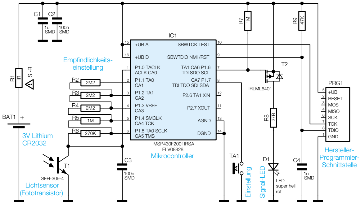
Bild 6: Das Schaltbild des aktiven Katzenauges AKA 100
