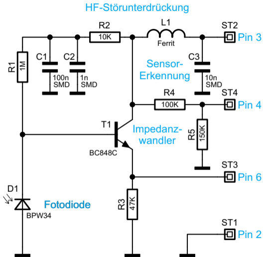
Bild 2: Schaltbild des ESA1000WZ-LED
