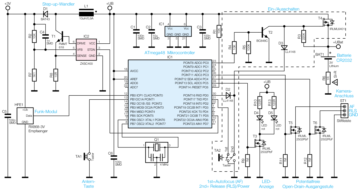
Bild 13: Das Schaltbild des FS20 FA
