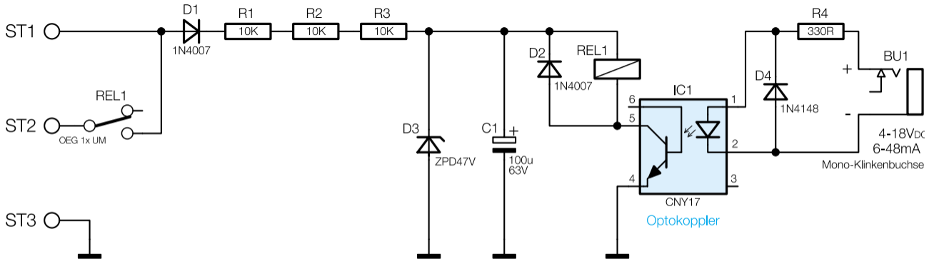
Bild 1: Schaltbild des 230-V-Schaltinterfaces SI 230-2
