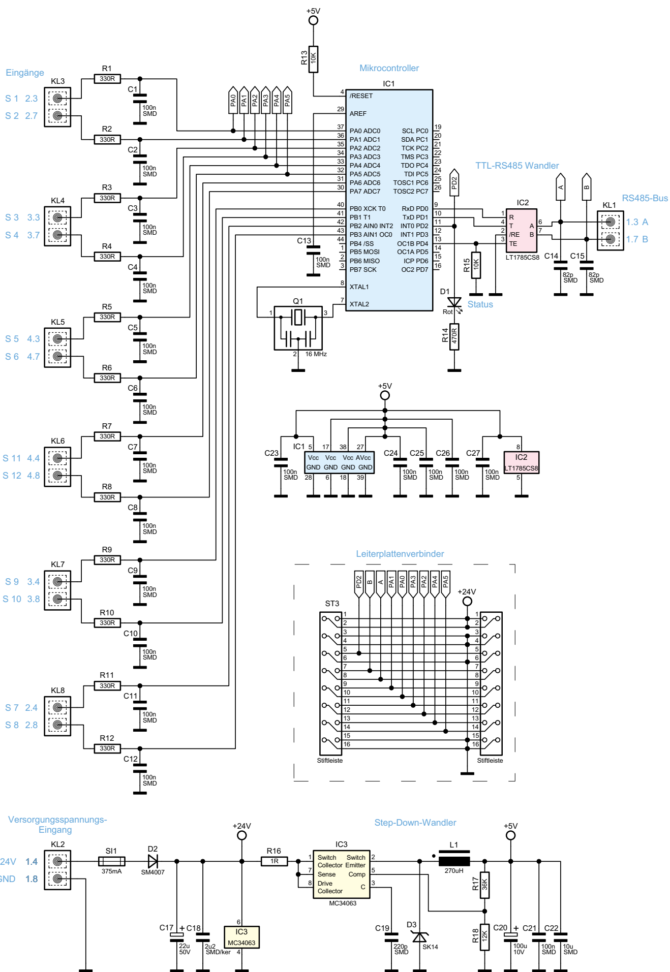
Bild 9: Schaltbild des HMW-Sen-SC-12-DR
