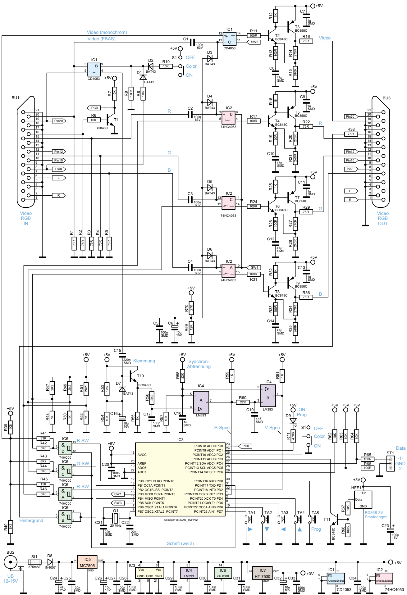
Bild 3: Das Schaltbild der FS20 OSD
