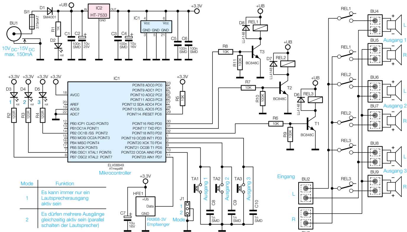
Bild 3: Die Schaltung des FS20-Lautsprecherumschalters
