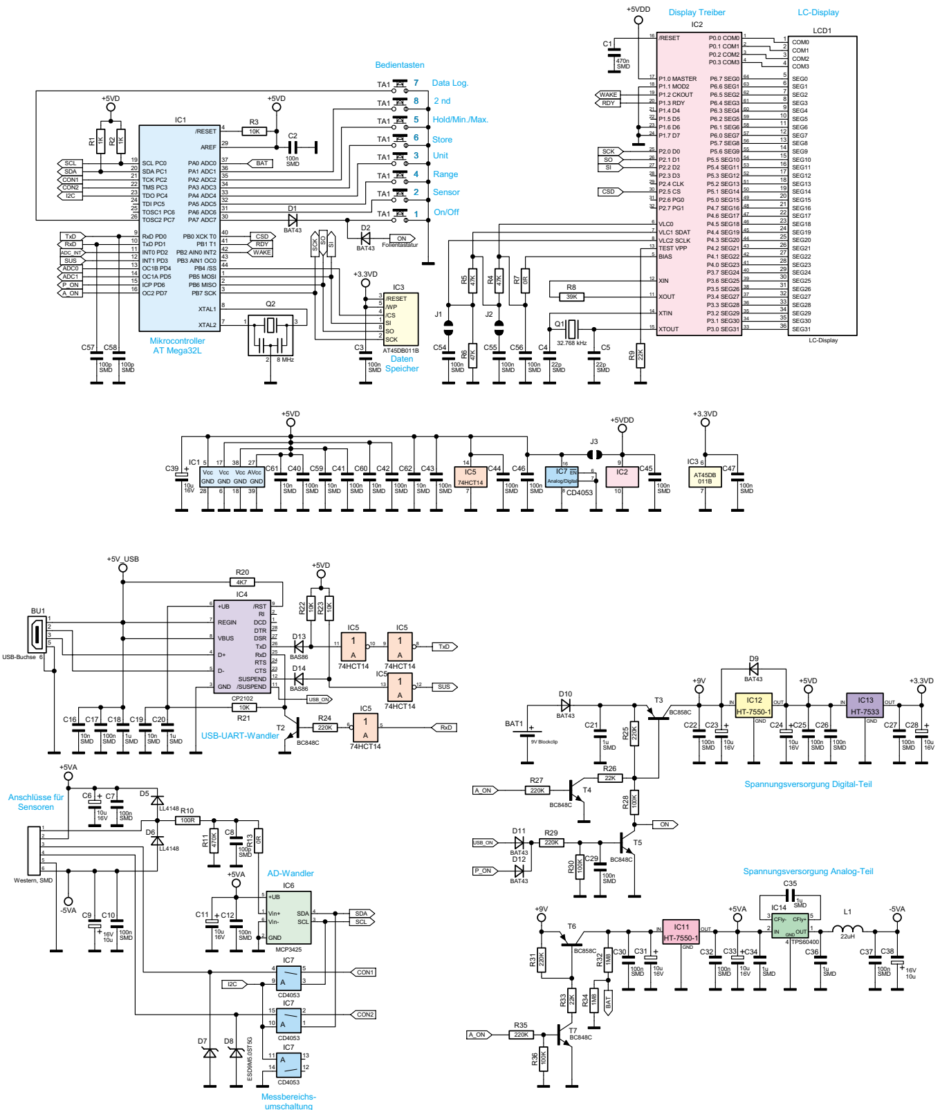
Bild 1: Die Schaltung des ULM 500, unterteilt in Spannungversorgung, USB-Schnittstelle, Sensor-Schnittstelle und Prozessorteil mit Datenspeicher und Displaysteuerung
