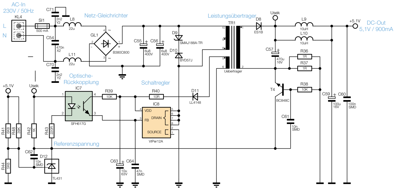
Bild 7: Das primär getaktete Schaltnetzteil mit <0,4 W Stand-by-Verbrauch
