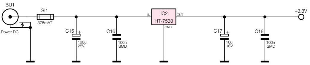
Bild 4: Hauptschaltbild der Mikrofon-Nebengeräusch-Unterdrückung
