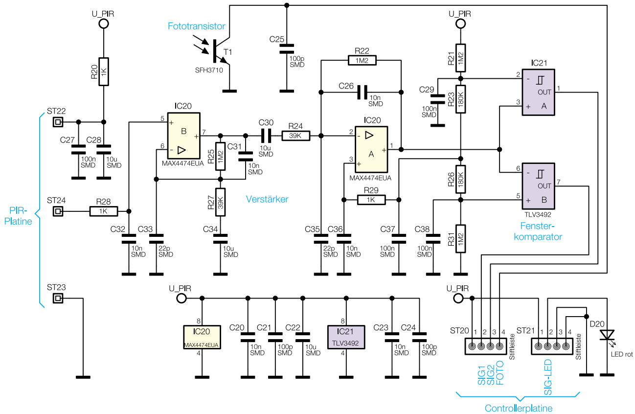
Bild 3: Die Schaltung, die auf der Frontplatte untergebracht ist: Verstärker, Komparator, Helligkeitssensor und Status-LED
