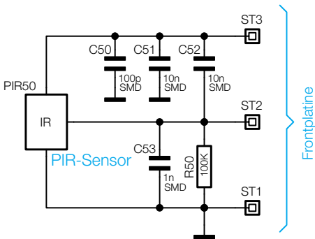
Bild 2: Der Schaltungsteil „PIR-Sensor“, der sich auf der PIR-Platine befindet
