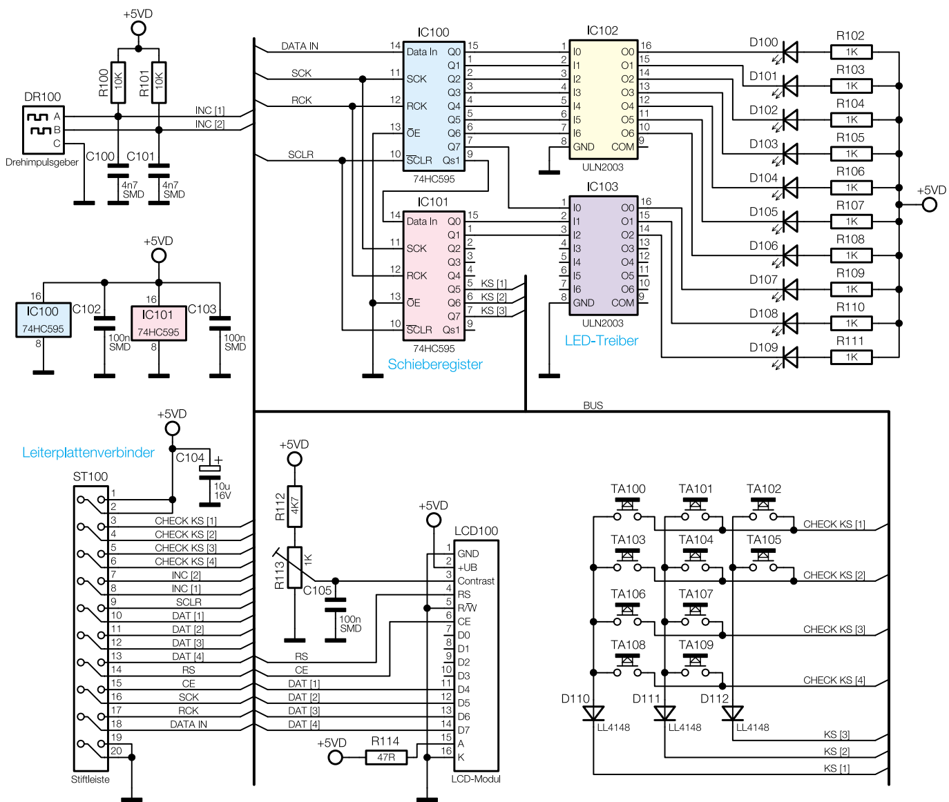
Bild 4: Schaltbild der Bedien- und Anzeigeeinheit (Frontplatte)
