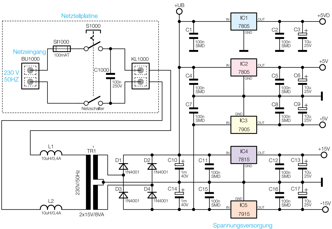
Bild 5: Schaltbild des Netzteils des DDS 8010
