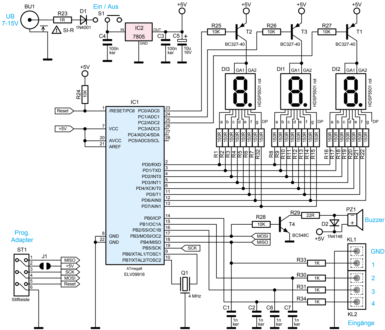
Bild 1: Schaltbild der Elektronik
