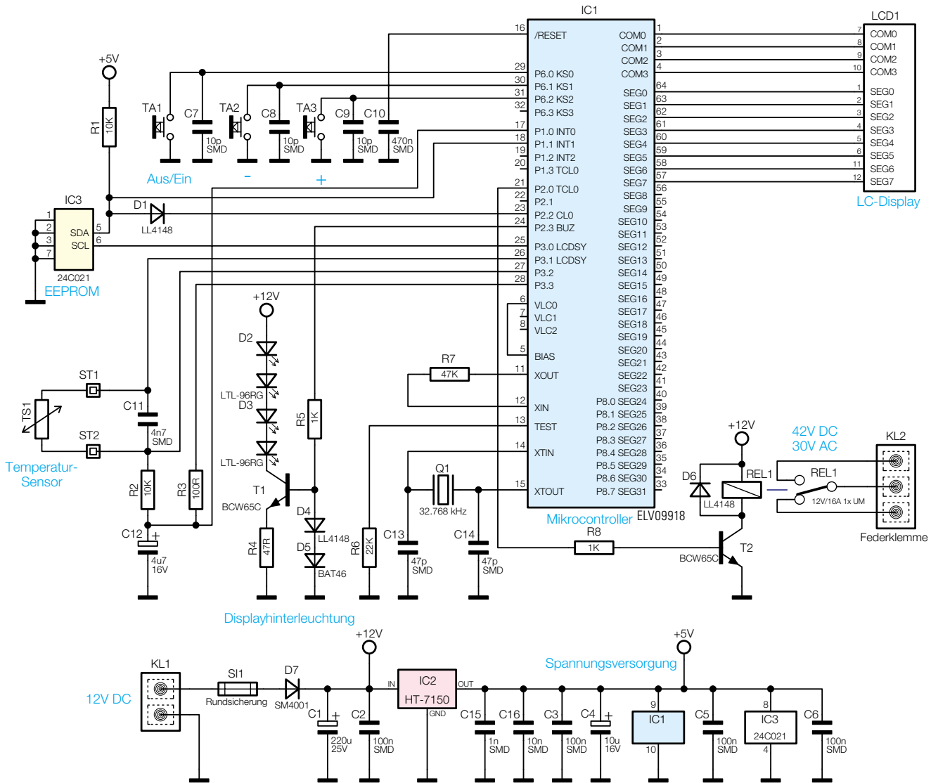
Bild 1: Das Schaltbild des UTM 200
