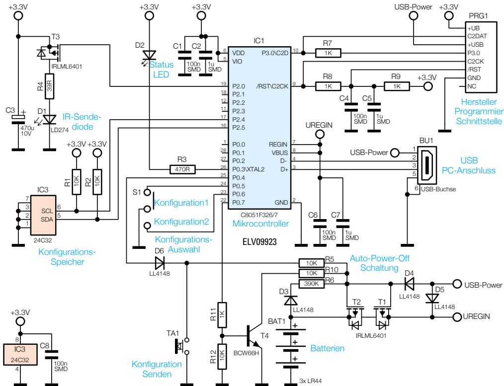
Bild 4: Die Schaltung des FS20 IRP2
