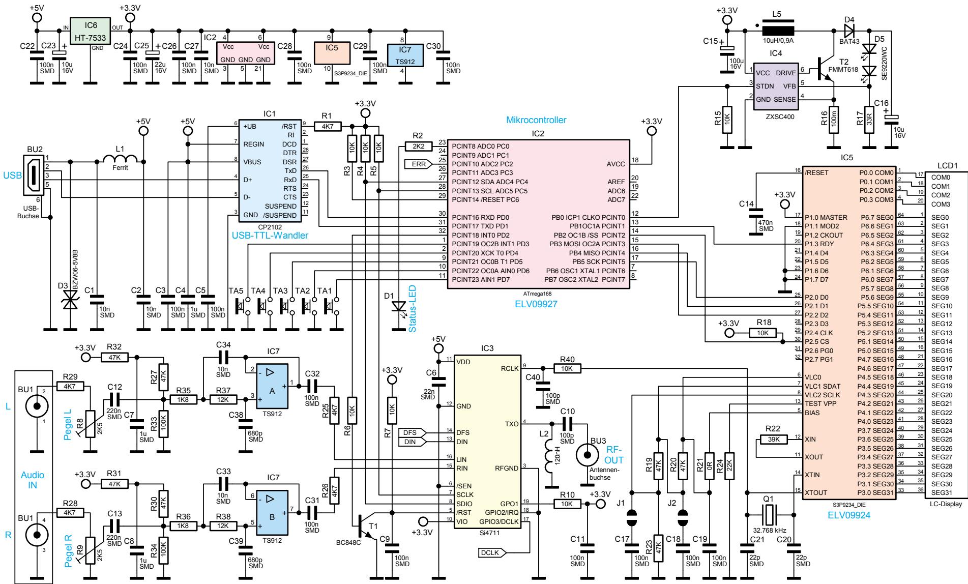
Bild 6: Das Hauptschaltbild des RDS-Stereo-Prüfgenerators SUP2
