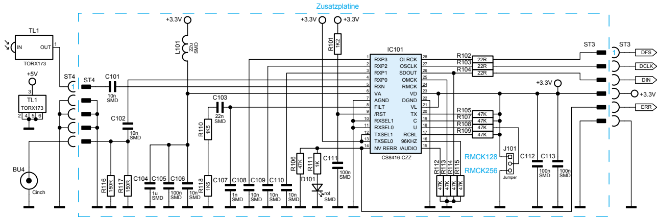
Bild 7: Die Schaltung der Digital-Audio-Zusatzschaltung
