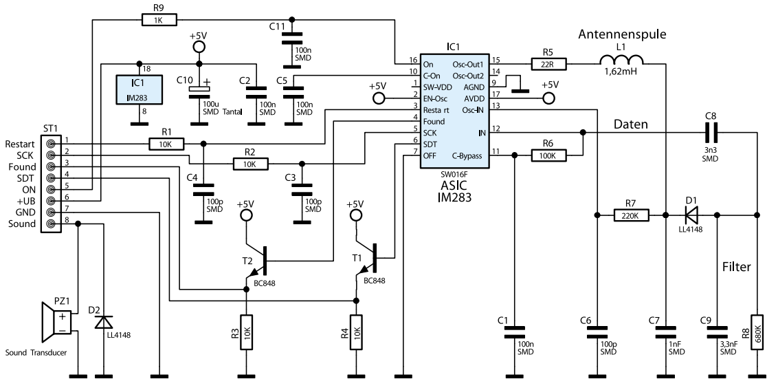
Bild 7: Schaltbild der Leseeinheit
