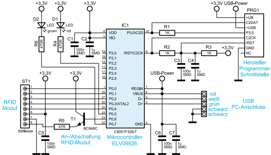
Bild 8: Schaltbild der Mikrocontrollereinheit
