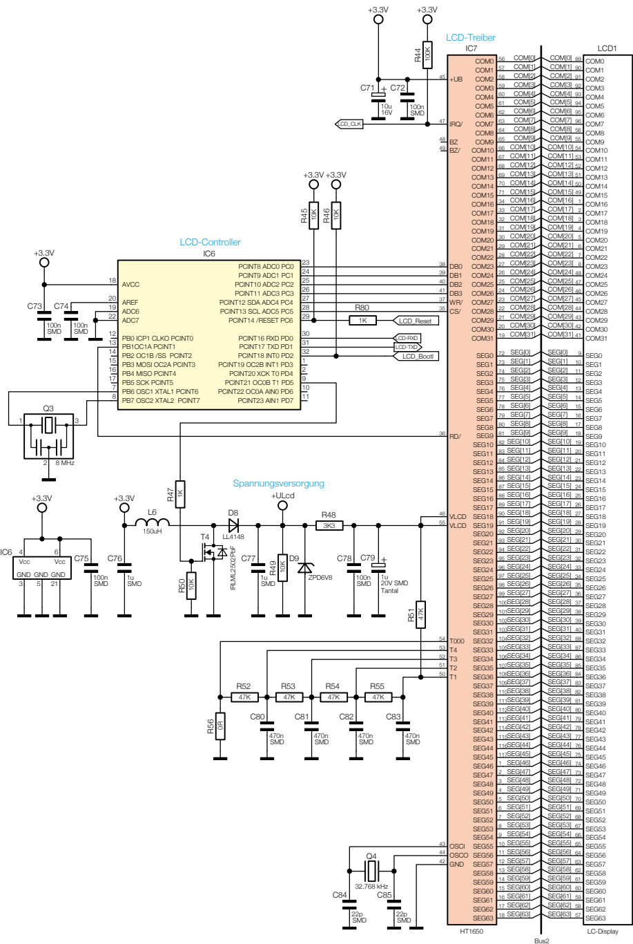
Bild 9: Die Schaltung der Displaysteuerung
