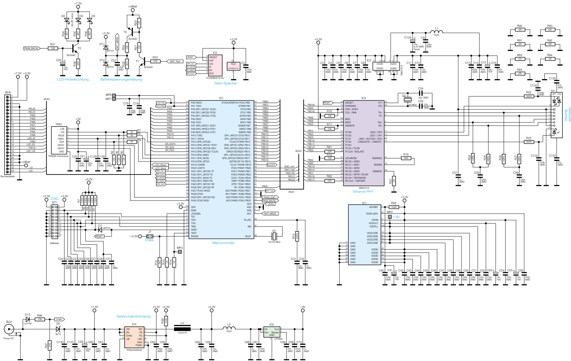
Bild 8: Die Schaltung der Steuerung der Alarmzentrale mit IC 1 als zentralem Element
